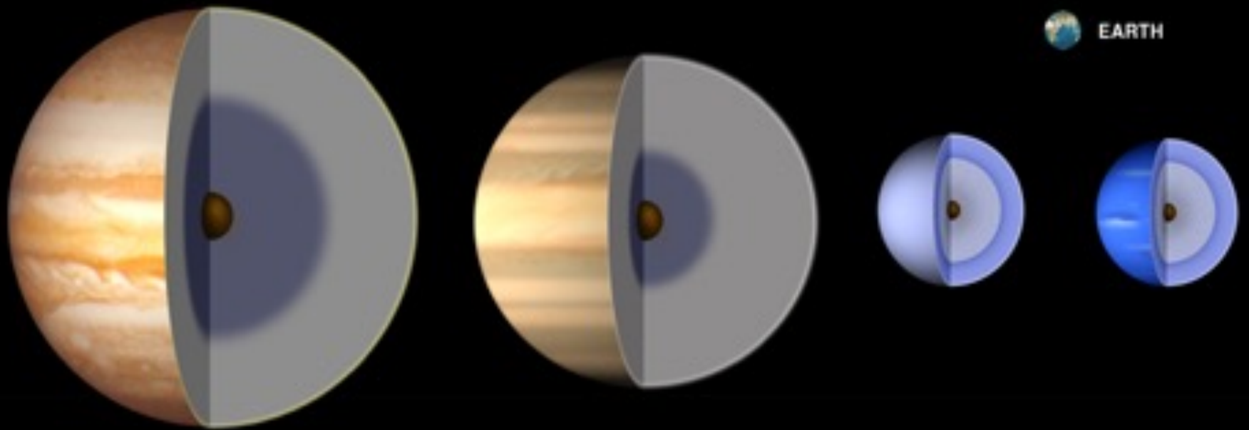
JUPITER
